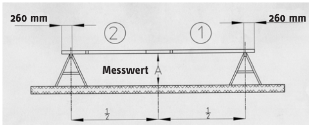
Bild 3: Unbelastete, umgesteckte Leiterteile
