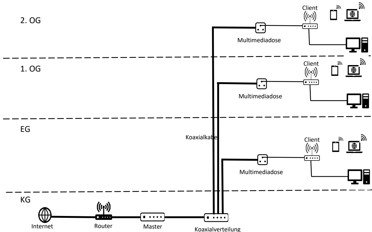
Abbildung 14: Koaxialnetzwerk
