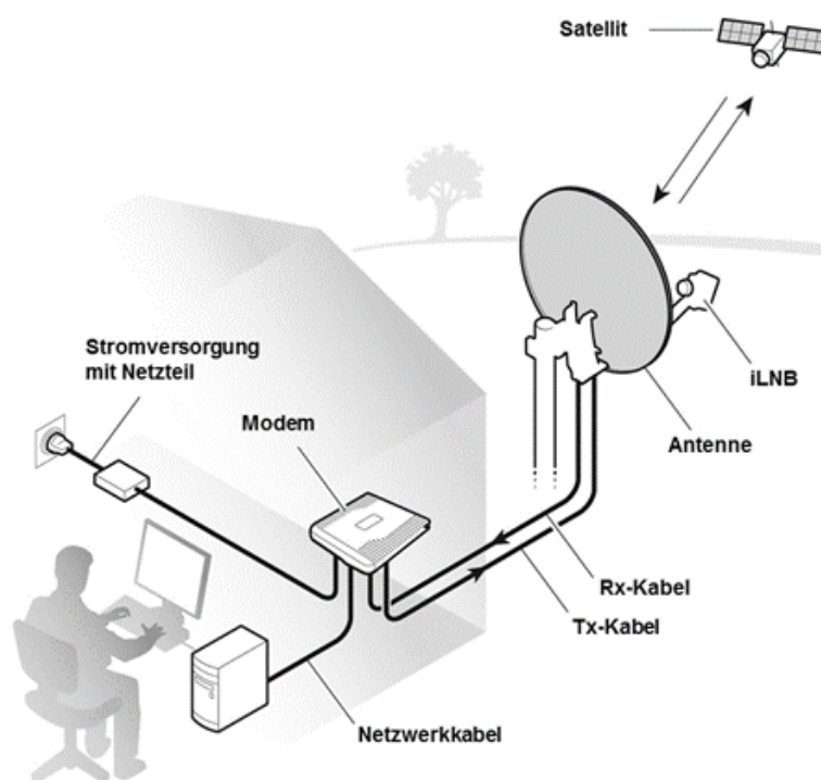
Abbildung 10: SAT-Internetanschluss
