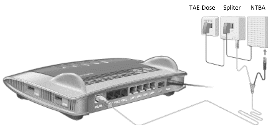
Abbildung 4: Router-Anschluss mit ISDN und NTB
