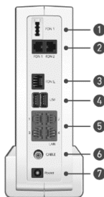
Abbildung 5: Kabelrouter-Anschlüsse
